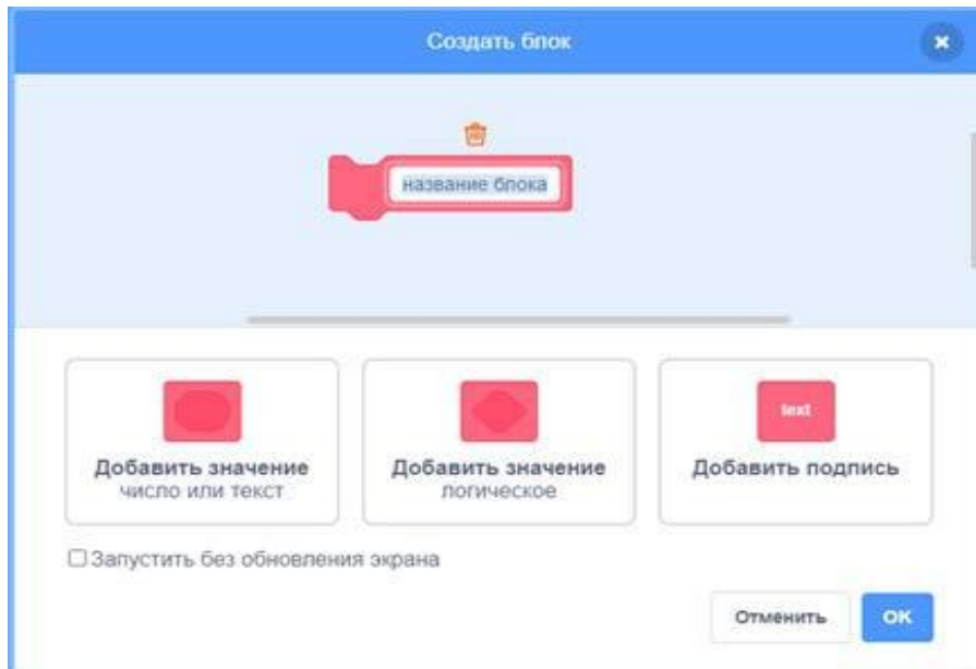
Рис. 133.. Вид диалогового окна для создания подпрограммы (нового блока)
